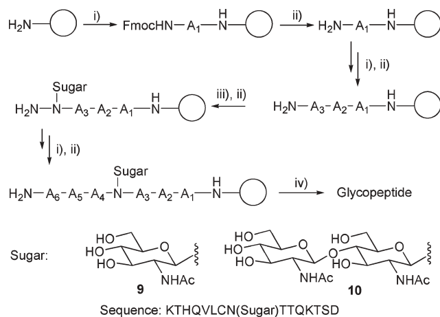
Scheme 3 i) Fmoc-A-OH, PyBOP, HOBt, DIEA, DMF, ii) 20% piperidine, DMF, iii) glycoamino acid, HATU, HOBt, DIEA, DMF, iv) TFA/TIS/H 2 O.
